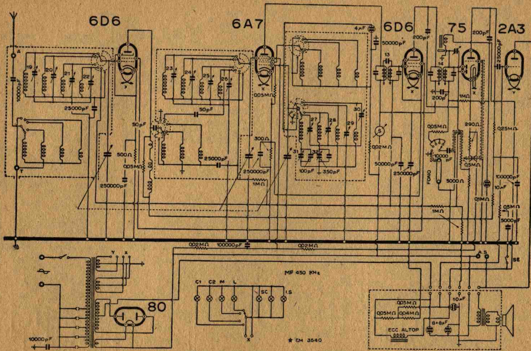
Lo schema elettrico del Quadri-Unda 637
